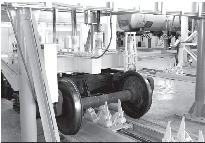
● Проектная мощность нового предприятия - 5000 вагоноремонтов в год.
