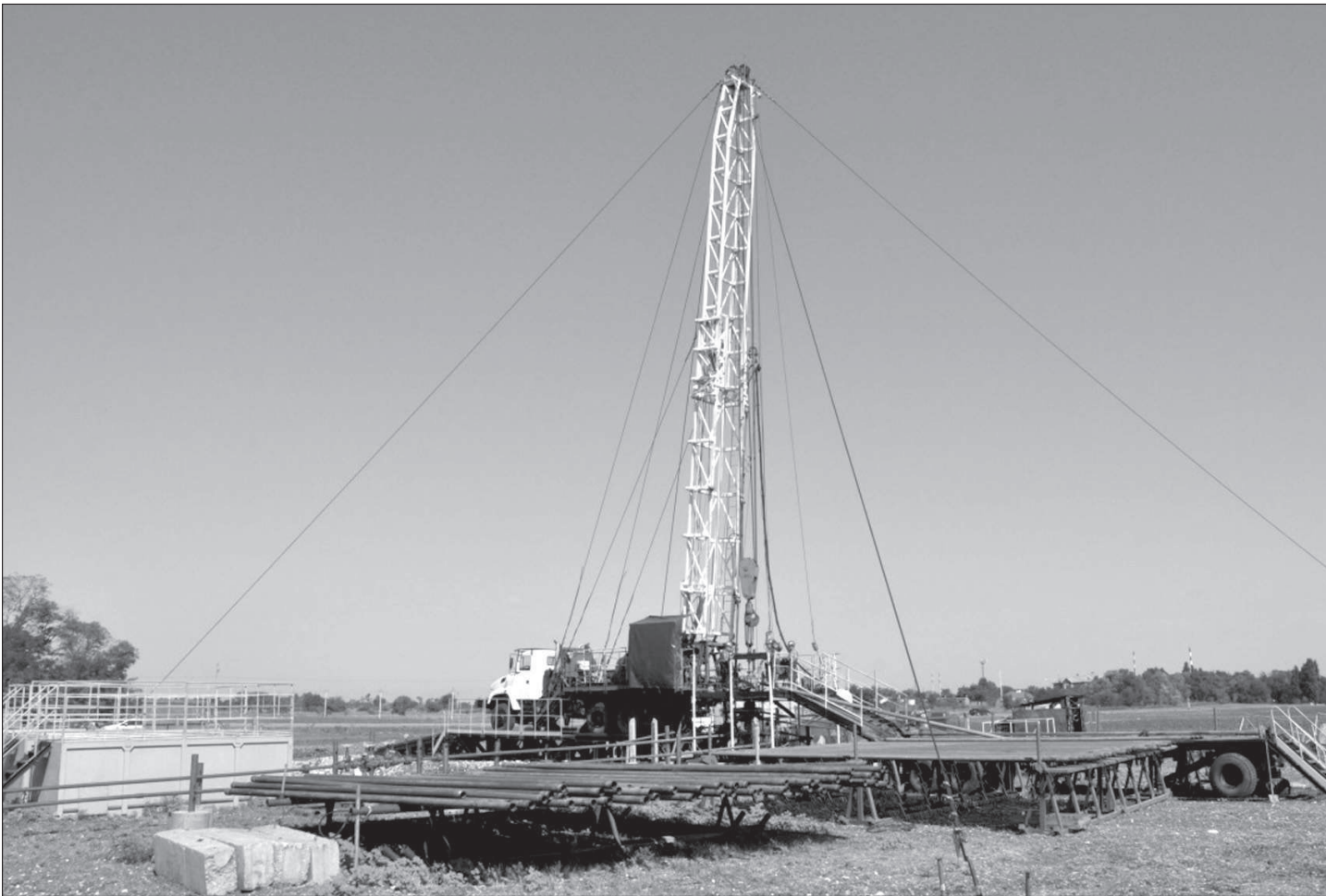
● Объекты Ставропольского управления аварийно-восстановительных работ и капитального ремонта скважин, филиала ООО «Газпром ПХГ».
